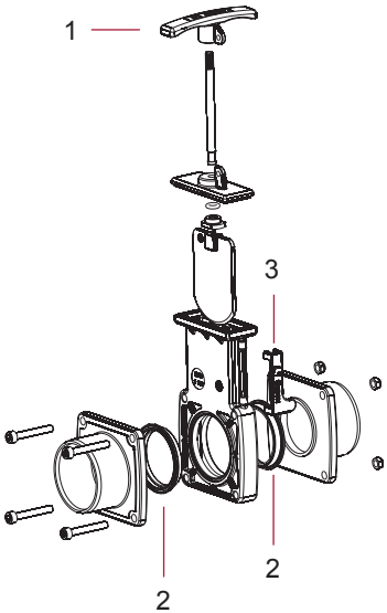
VALVOLE A GHIgliOTTINA IN PVC-U D50-D63
